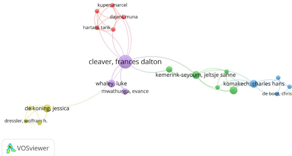
Gambar 4. Visualisasi Penulis
