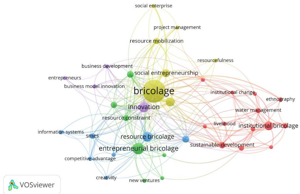
Gambar 1. Visualisasi Jaringan
