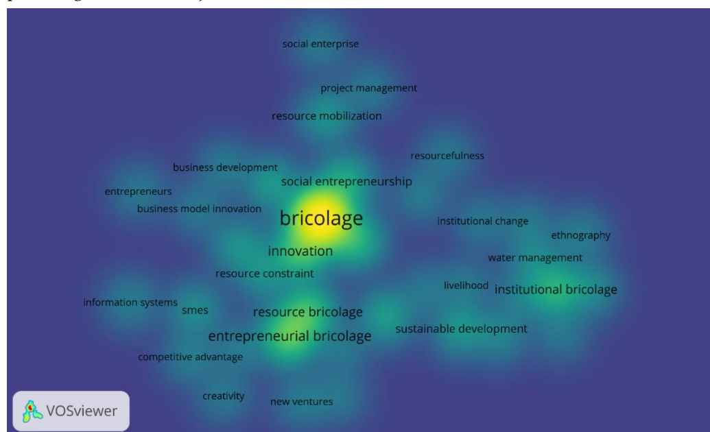
Gambar 3. Visualisasi Densitas
